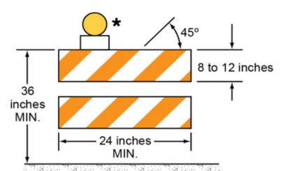
Type 2 Barricade
