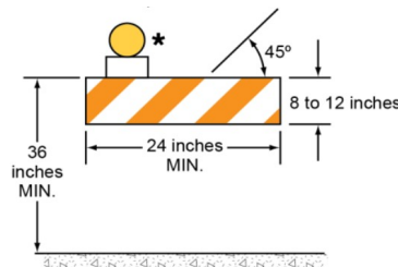
Type 1 Barricade
