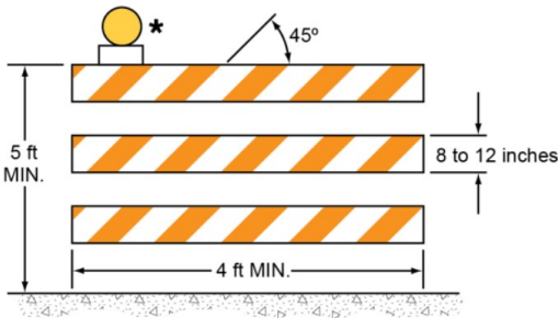
Type 3 Barricade
